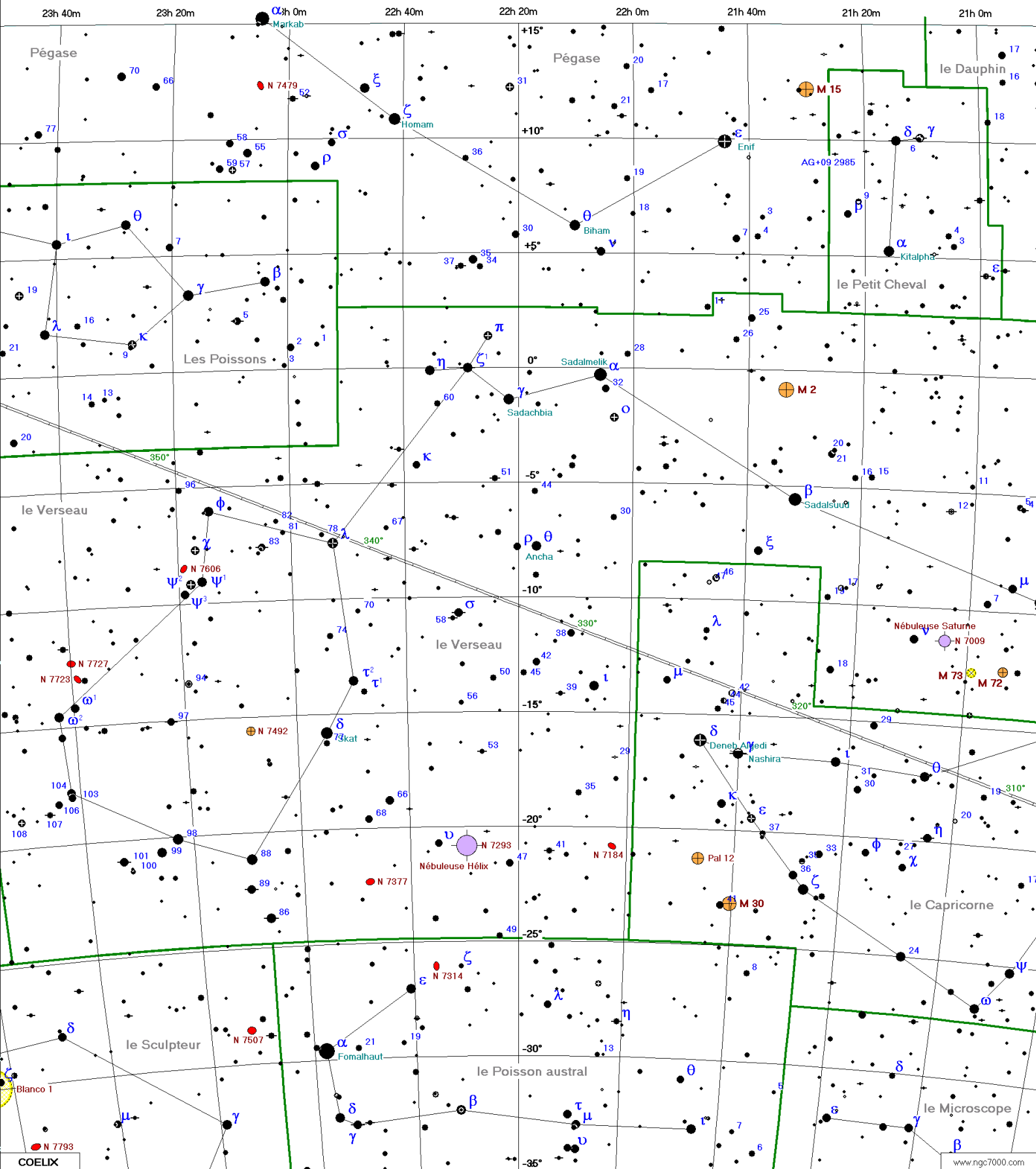
Magnitudes stellaires
